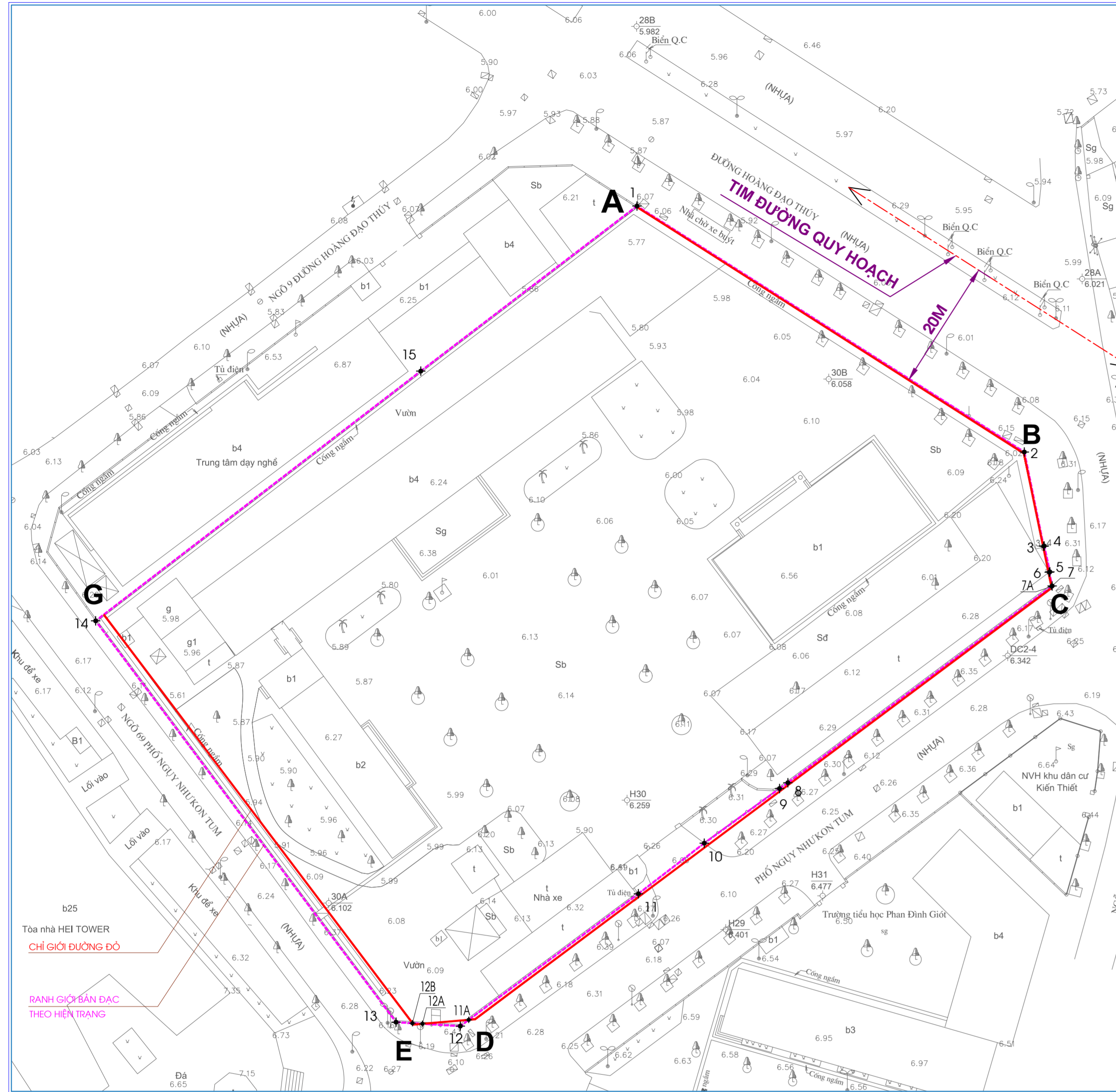
BẢN VẼ HIỆN TRẠNG VÀ CHỈ GIỚI ĐƯỜNG ĐỎ, TỶ LỆ 1/500
